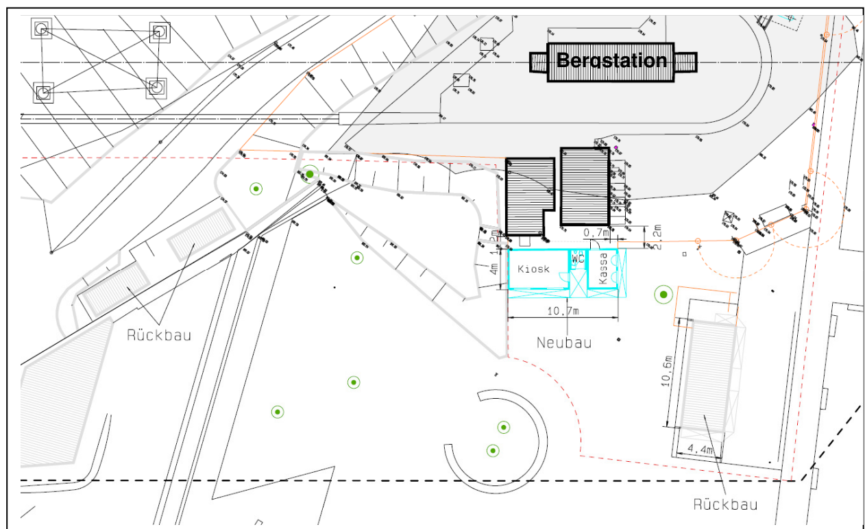
Abb. 10: Lageplanauszug Bergstation: Rückbau und Neubau von Containergebäude
