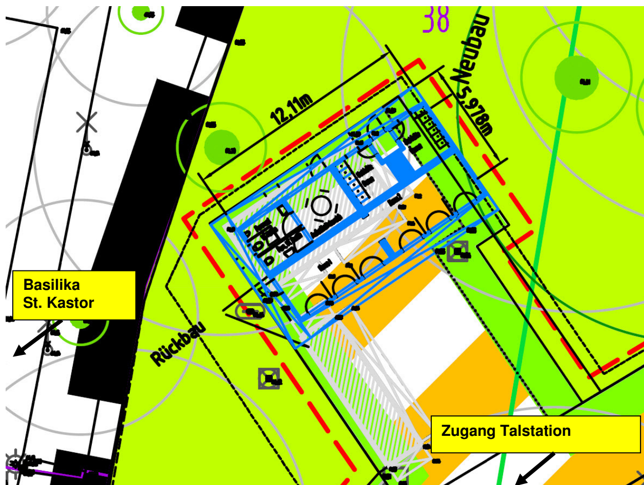
Abb. 7: Auszug Konzeption Bebauungsplan und überlagerter technischer Planung "Rückbau und Neubau von Containergebäuden"
