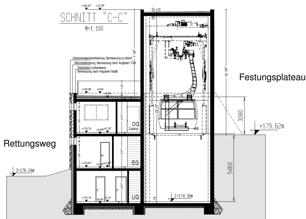
Abb. 12: Auszug Vorentwurfsplanung Doppelmayr (Stand 11/2013): Gebäudeschnitt Revisionsgebäude im Bereich Kabinenaufzug
