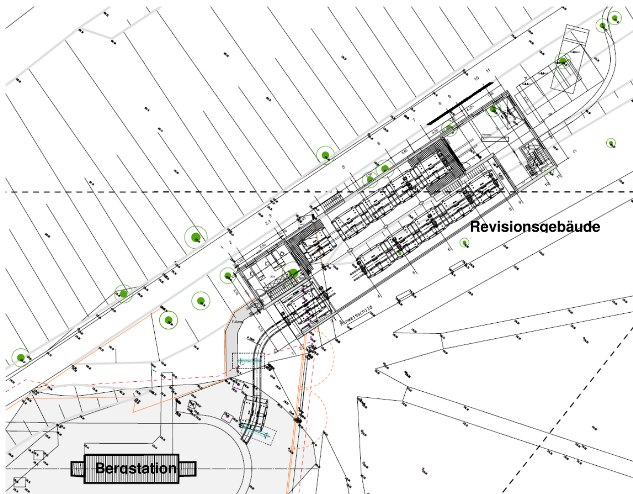
Abb. 11: Auszug Vorentwurfsplanung Doppelmayr (Stand 11/2013): Lageplanauszug Revisionsgebäude
