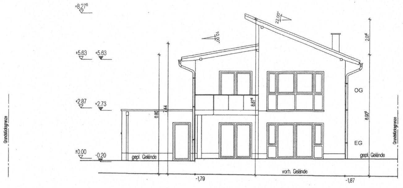
ANSICHT NORD - WEST
