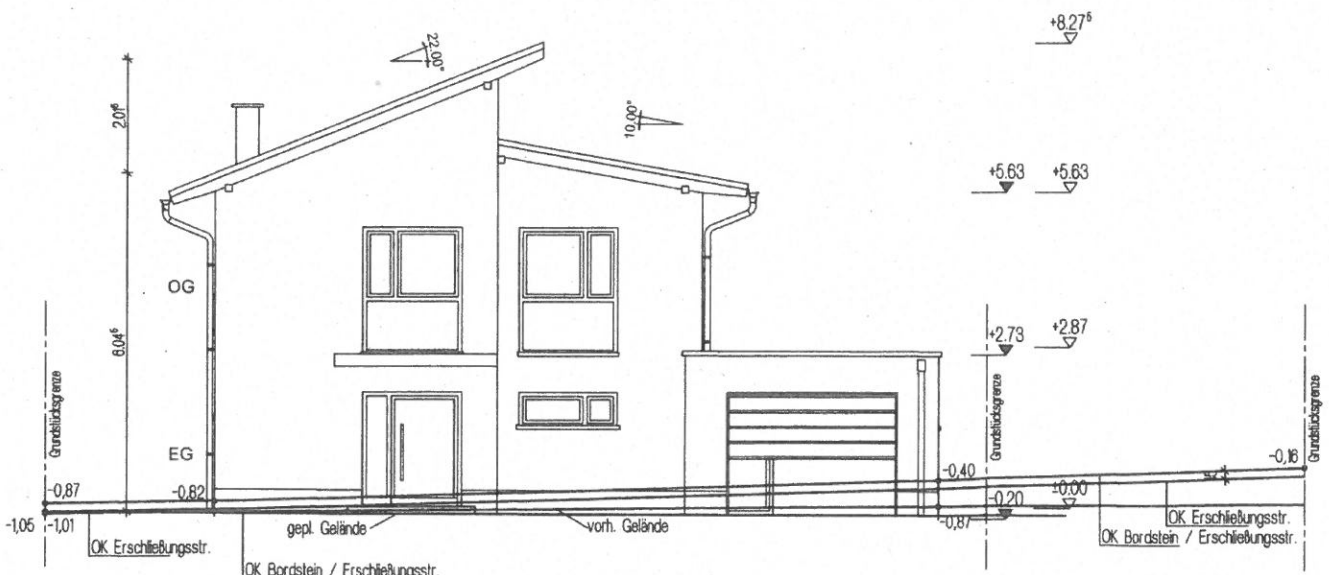
ANSICHT SÜD - OST
