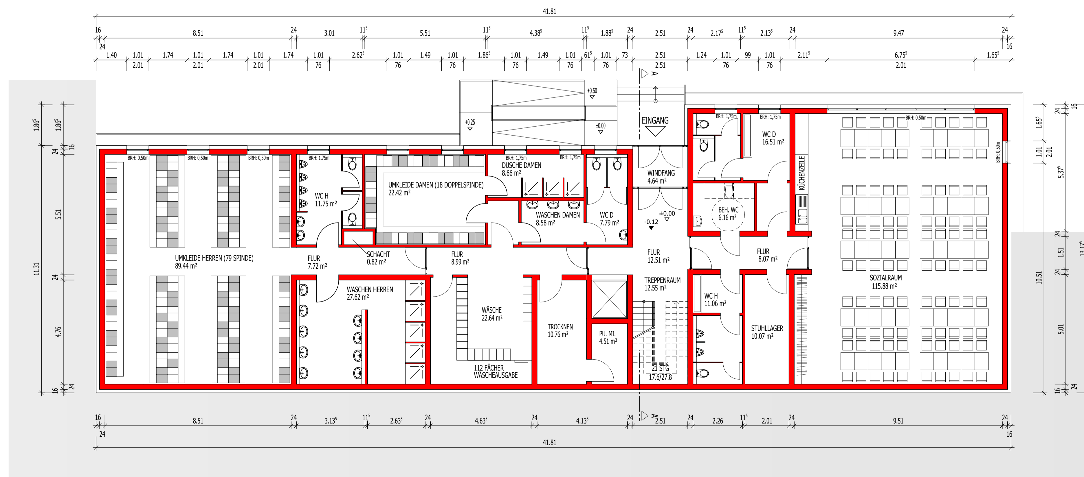
GRUNDRISS EG
