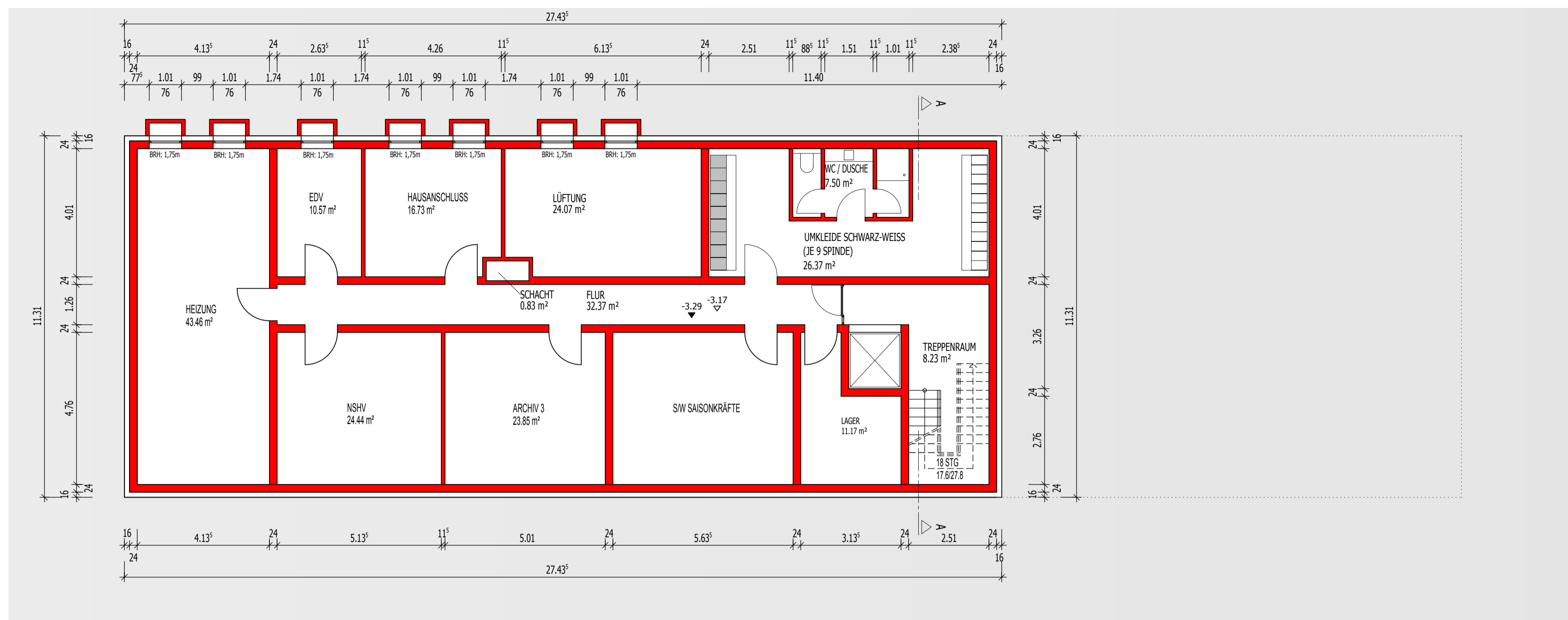
GRUNDRISS KG
