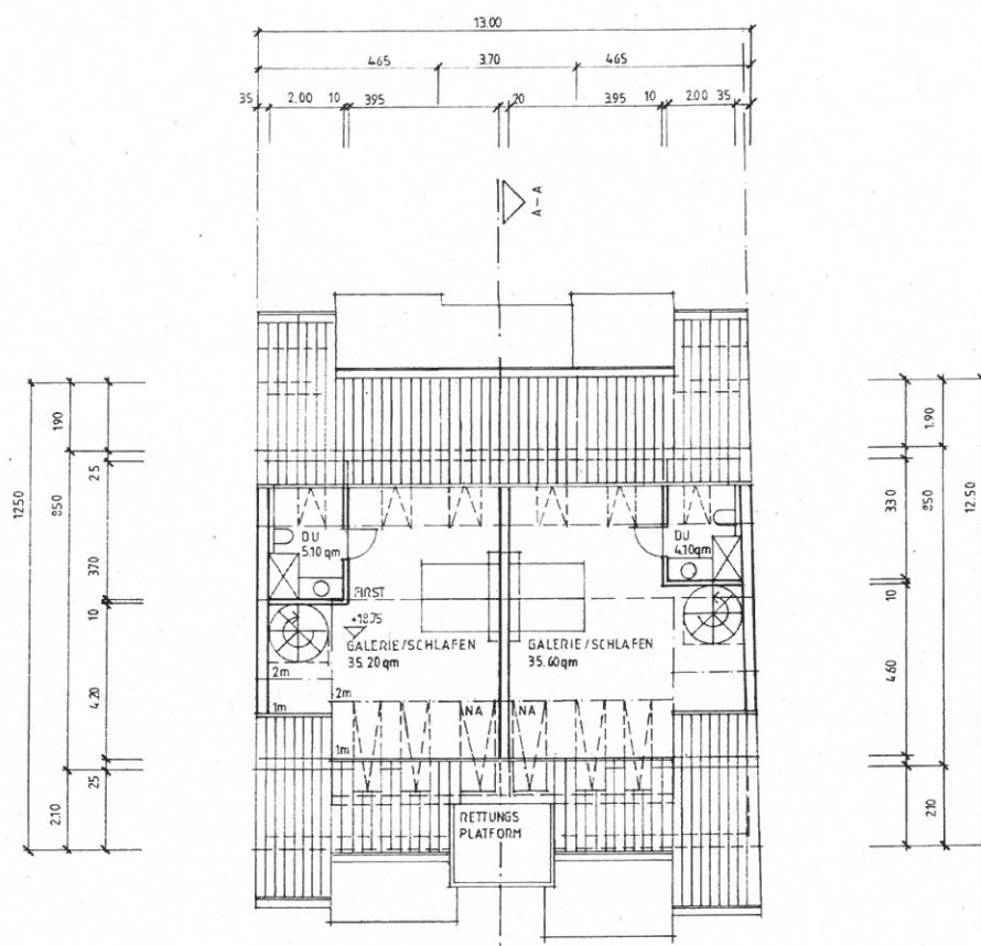
GRUNDRISS GG
