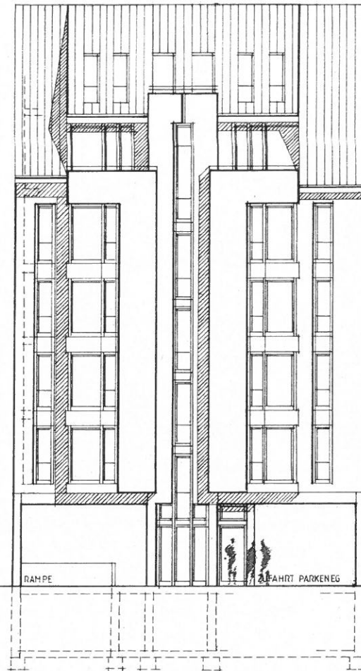
ANSICHT WESTEN ANDERNACHER STRASSE NR.22
