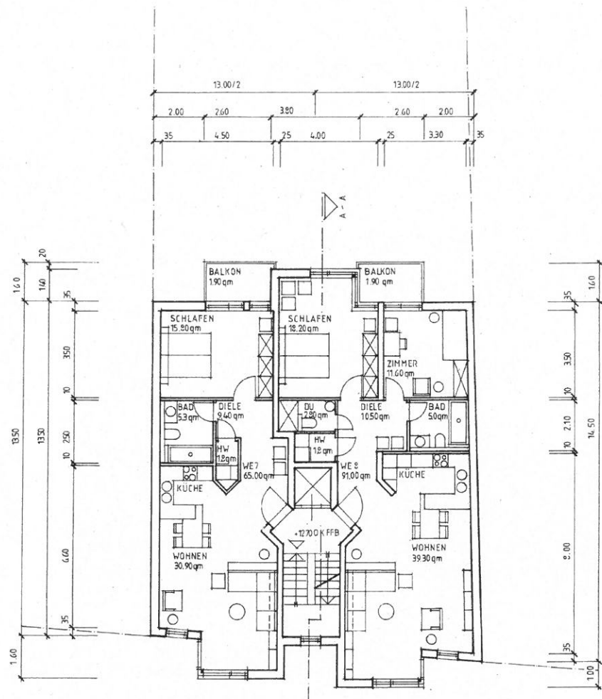
GRUNDRISS OG IV
