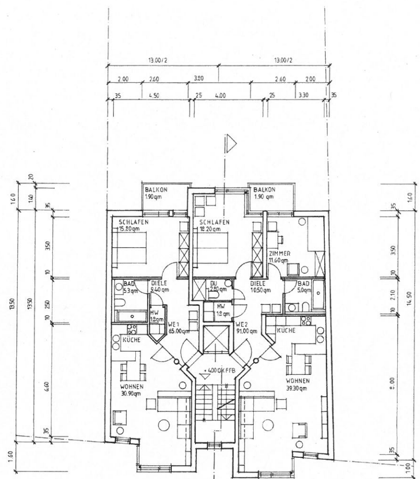
GRUNDRISS OG I
