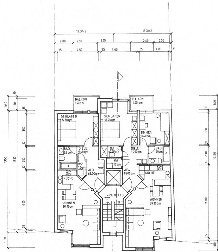
GRUNDRISS OG II
