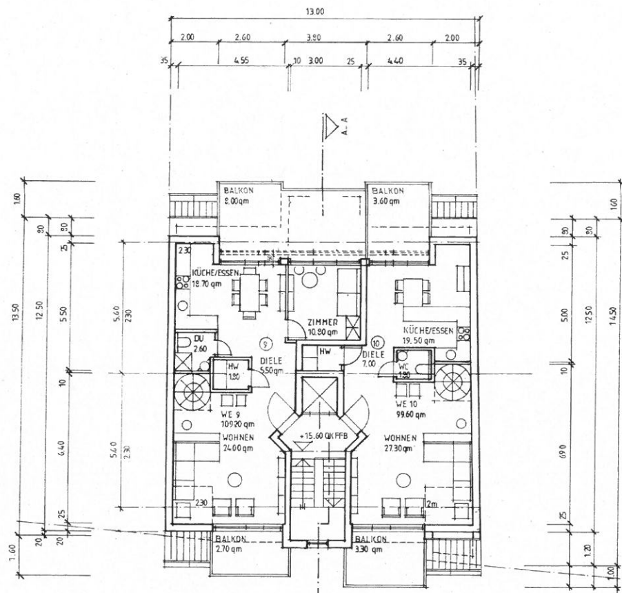
GRUNDRISS DG
