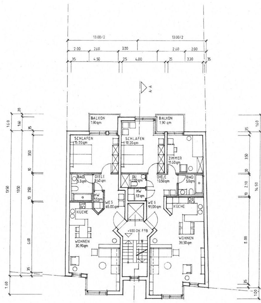
GRUNDRISS OG III
