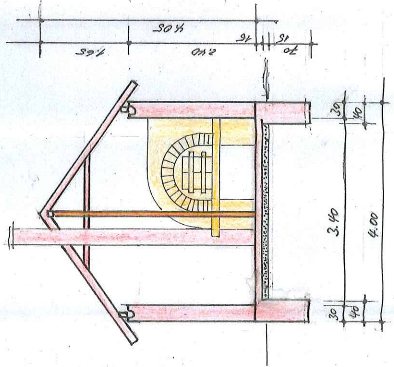
SCHNITT
