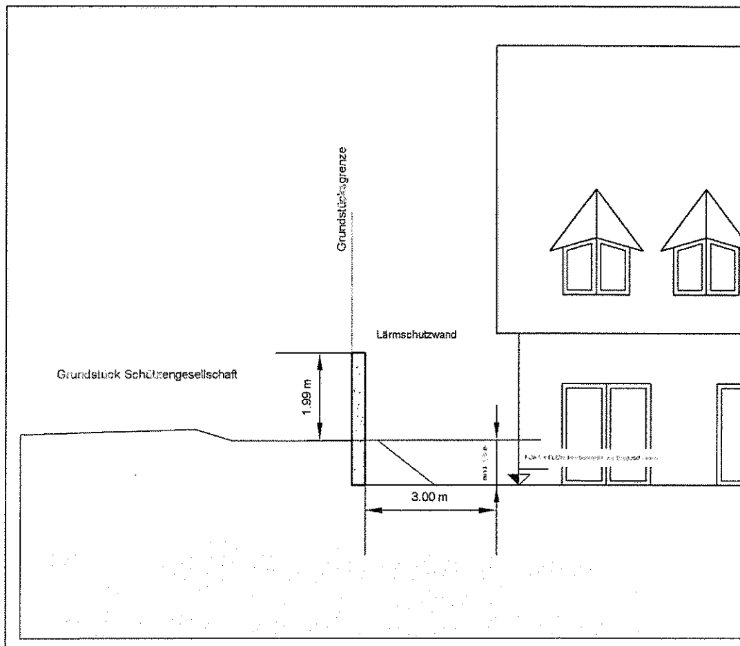
Abb.6 : System-Skizze Lärmschutzwand
