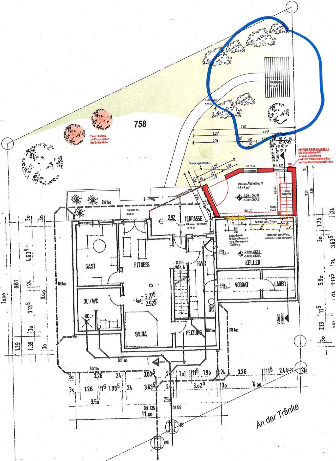
KELLERGESCHOSS PLANUNG
