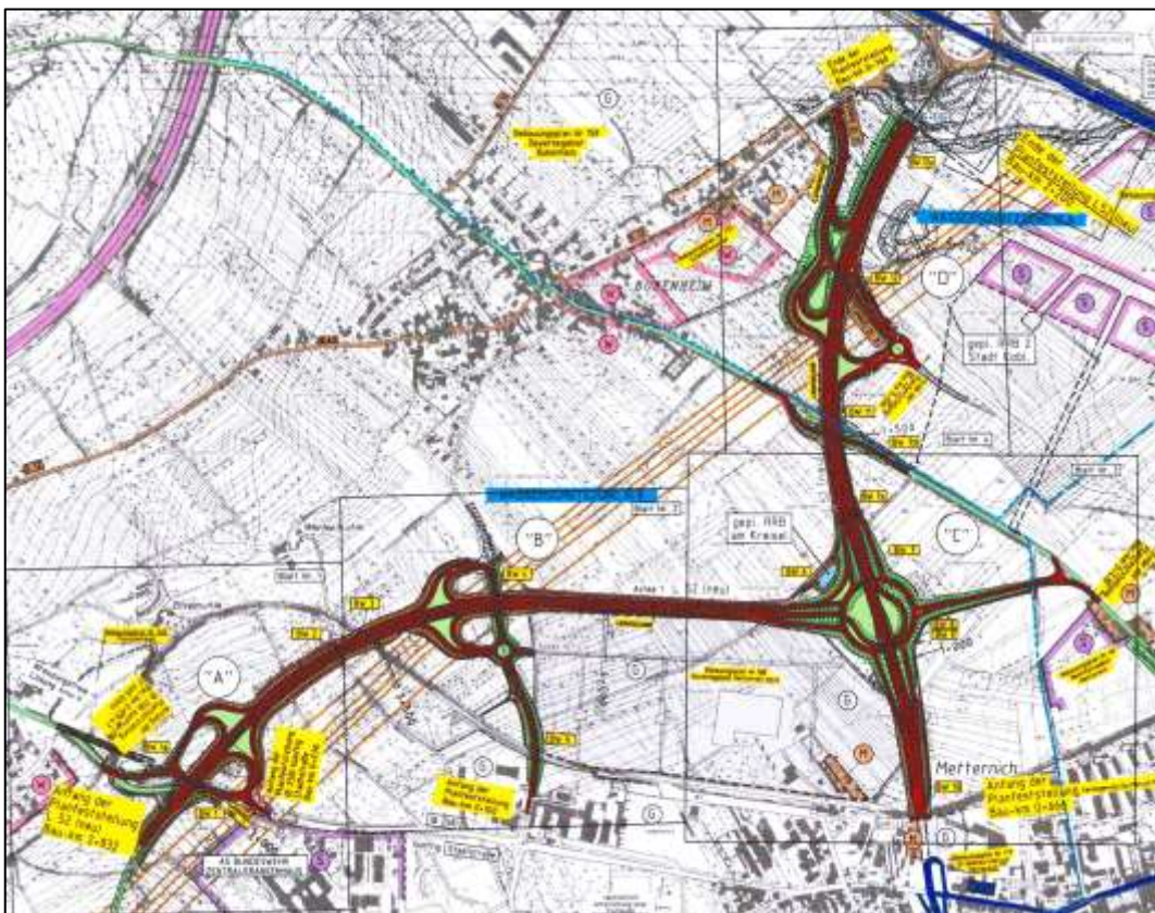
Abb. 22: Übersichtsplan aus der Planfeststellung Nordtangente
