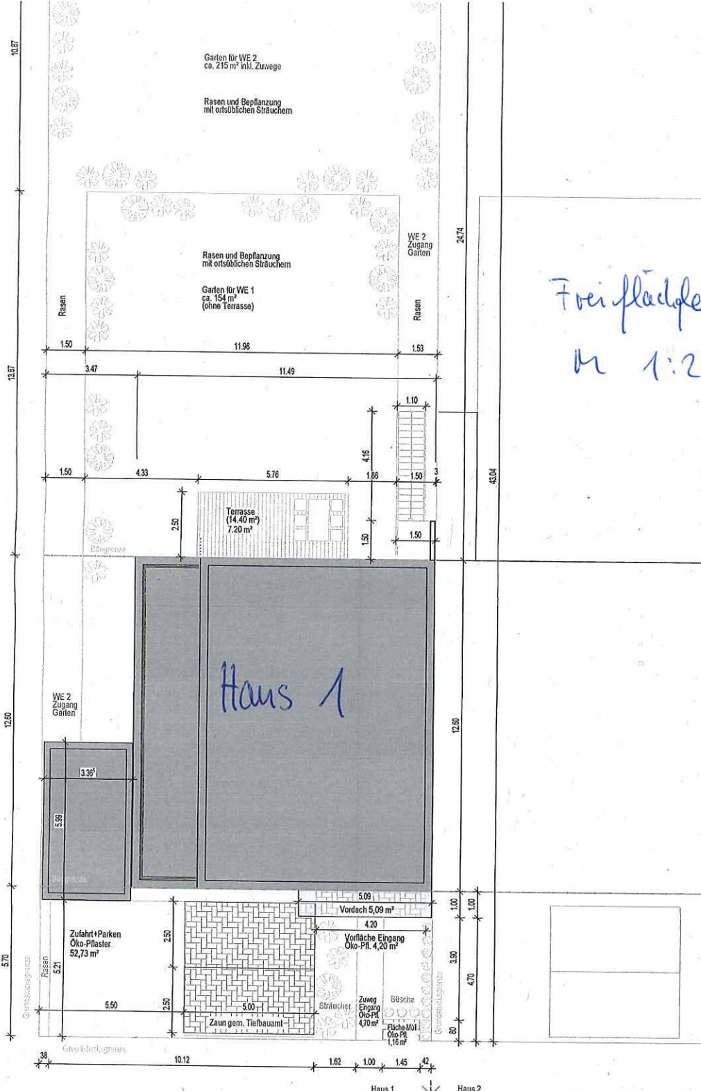
Freiflächenplan
