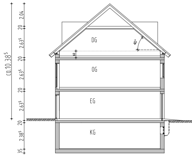
Schemaschnitt A-A
