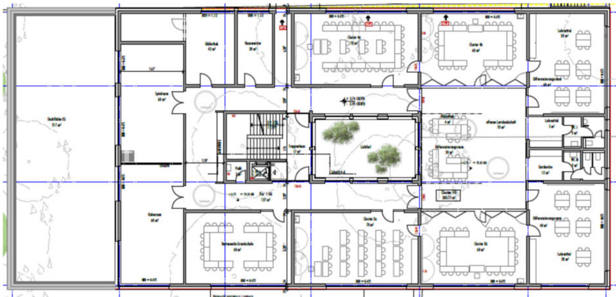
Abbildung 4: Grundriss OG
