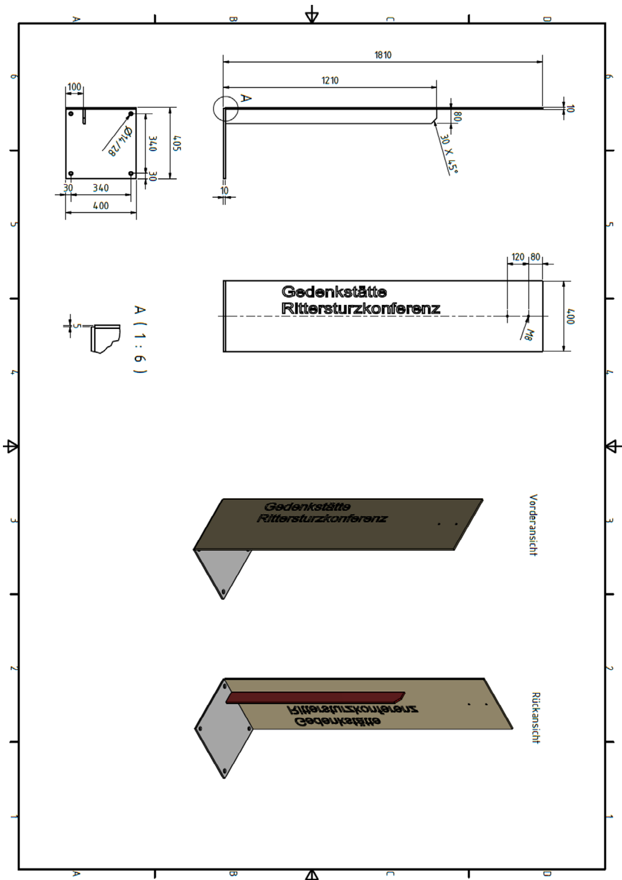
Abbildung 3: Entwurf Schild aus Cortenstahl
