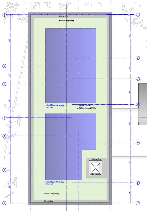
Abbildung 3: Grundriss DG
