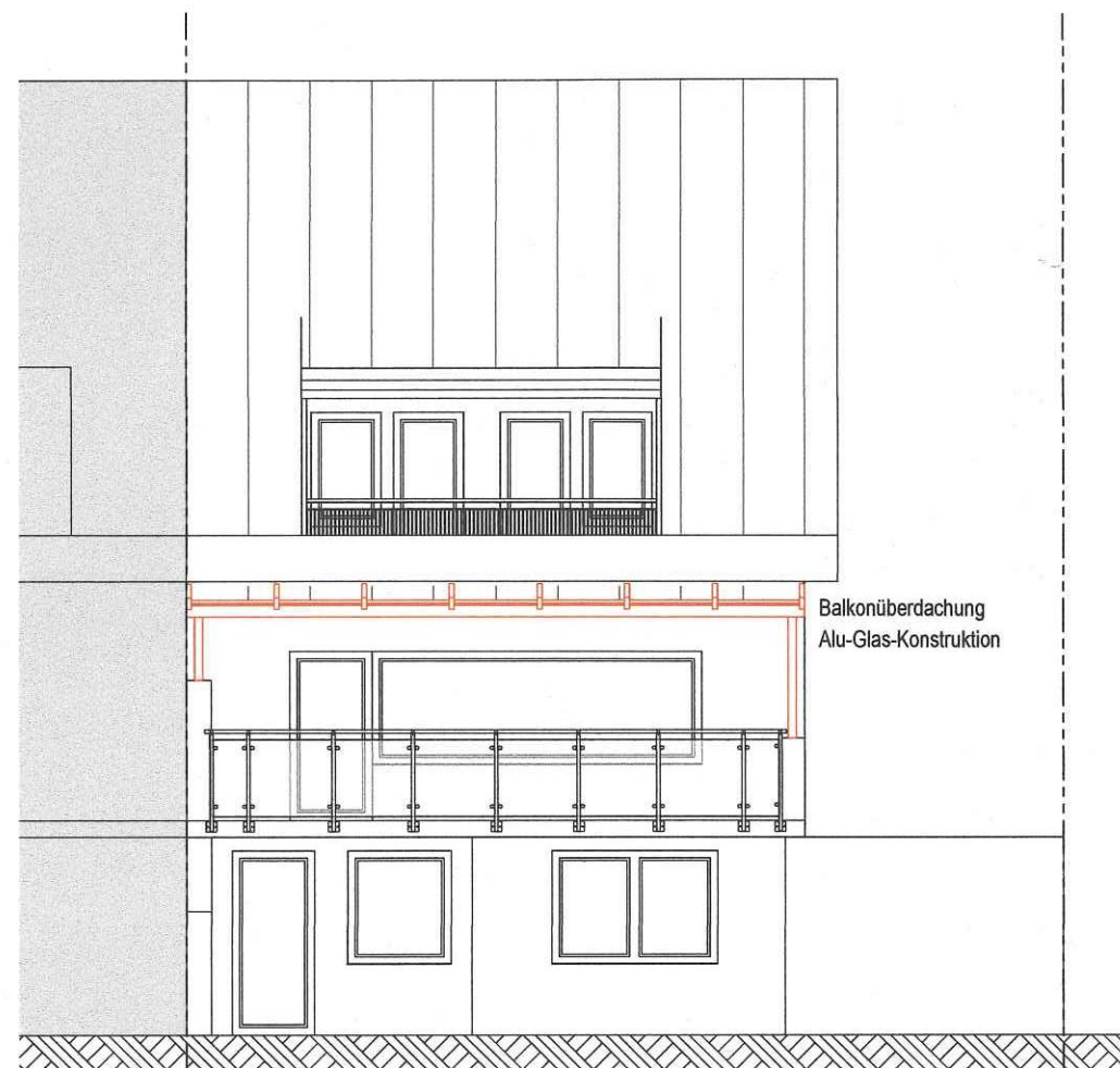
Ansicht Norden
