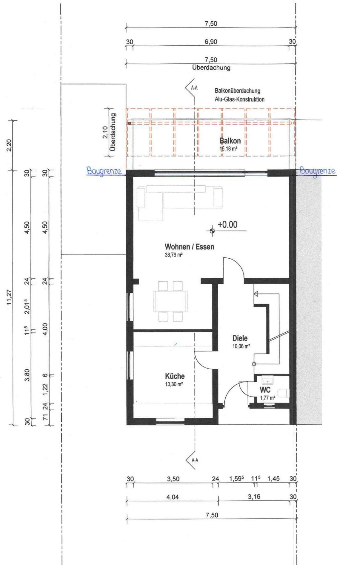
Erdgeschoss
