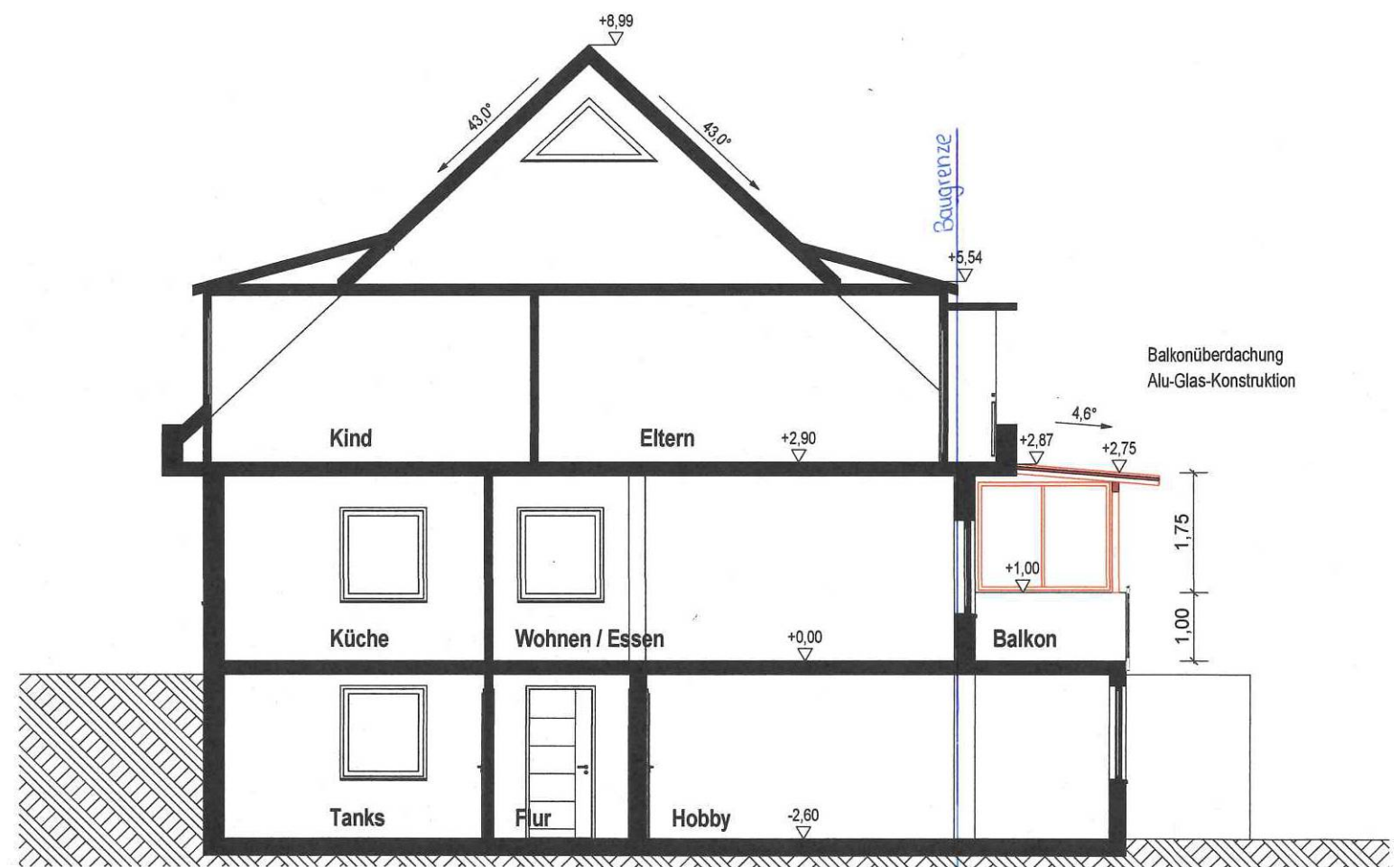
Schnitt A-A
