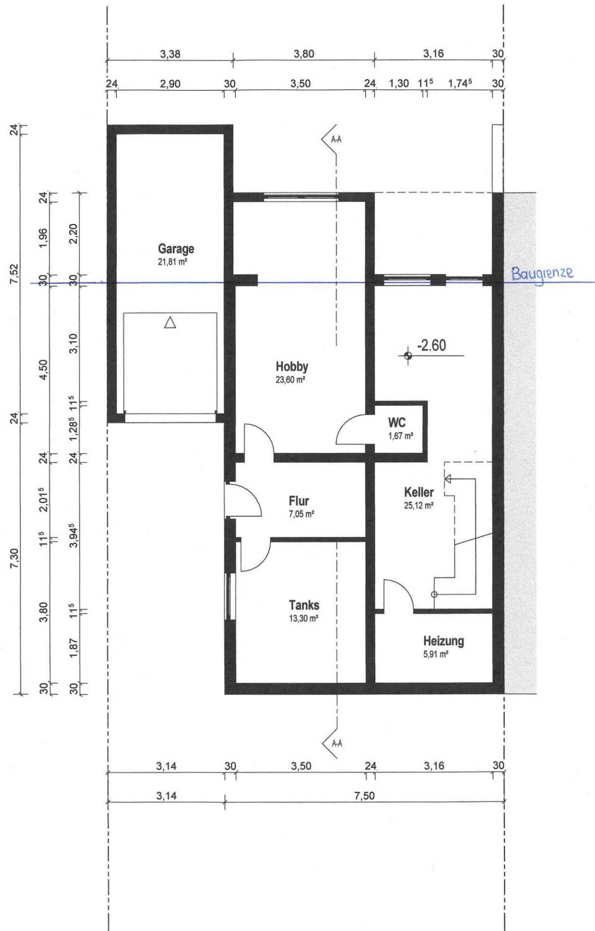
Kellergeschoss
