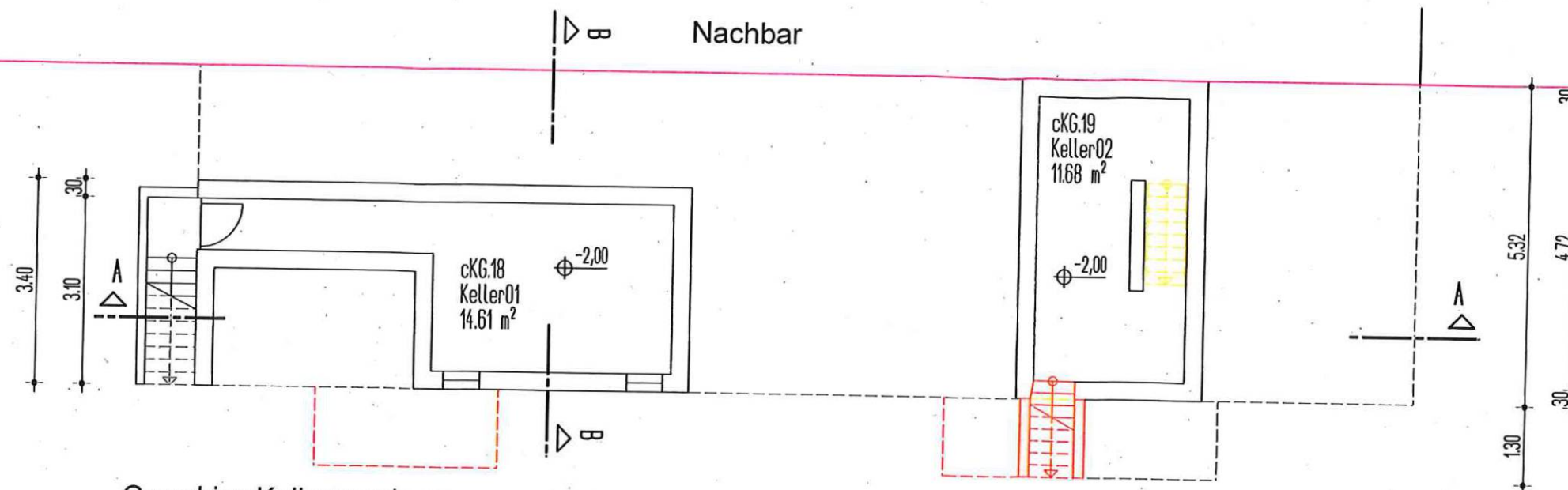
Grundriss Kellergeschoss
